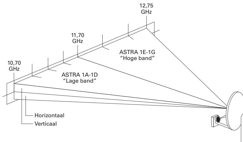
Ontvangst van de volledige ASTRA-frequentieband
